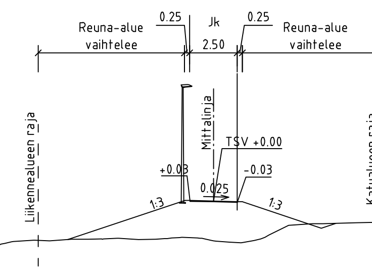
Maarinporras TYYPPIPOIKKILEIKKAUS G-G 1:200
