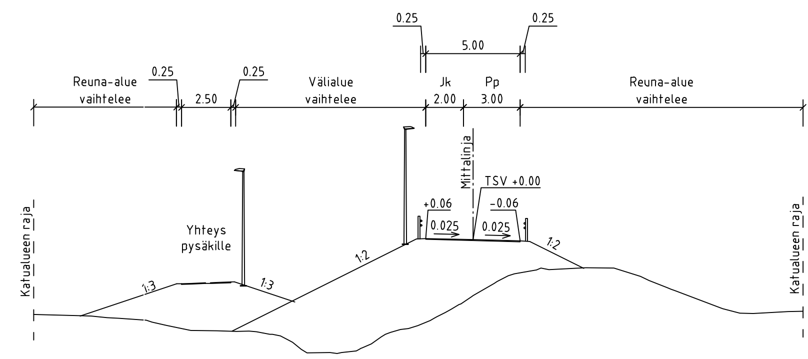
Maarinporras TYYPPIPOIKKILEIKKAUS E-E 1:200
