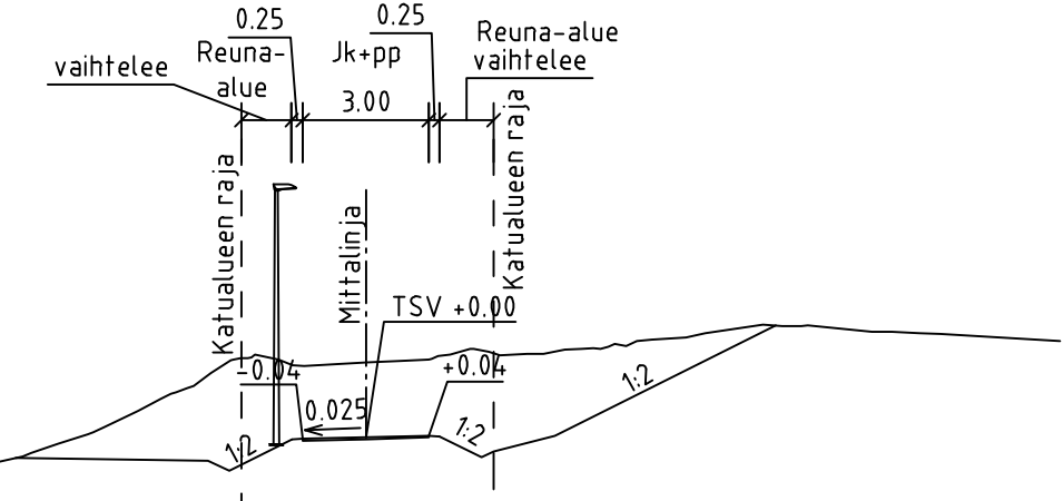
Metsänneidonpolku TYYPPIPOIKKILEIKKAUS H-H 1:200
