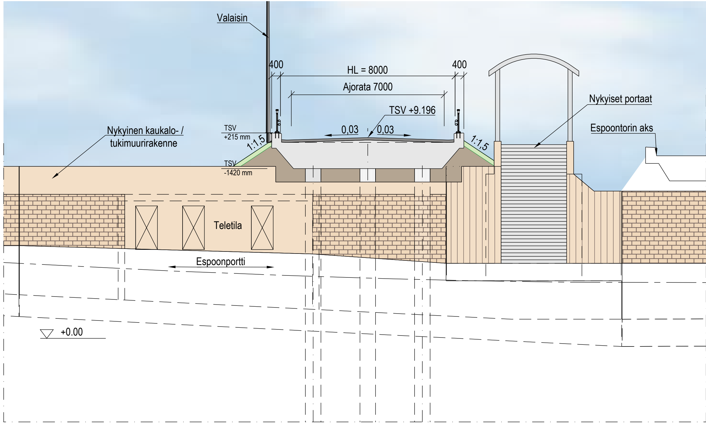
POIKKILEIKKAUS B - B 1:100
