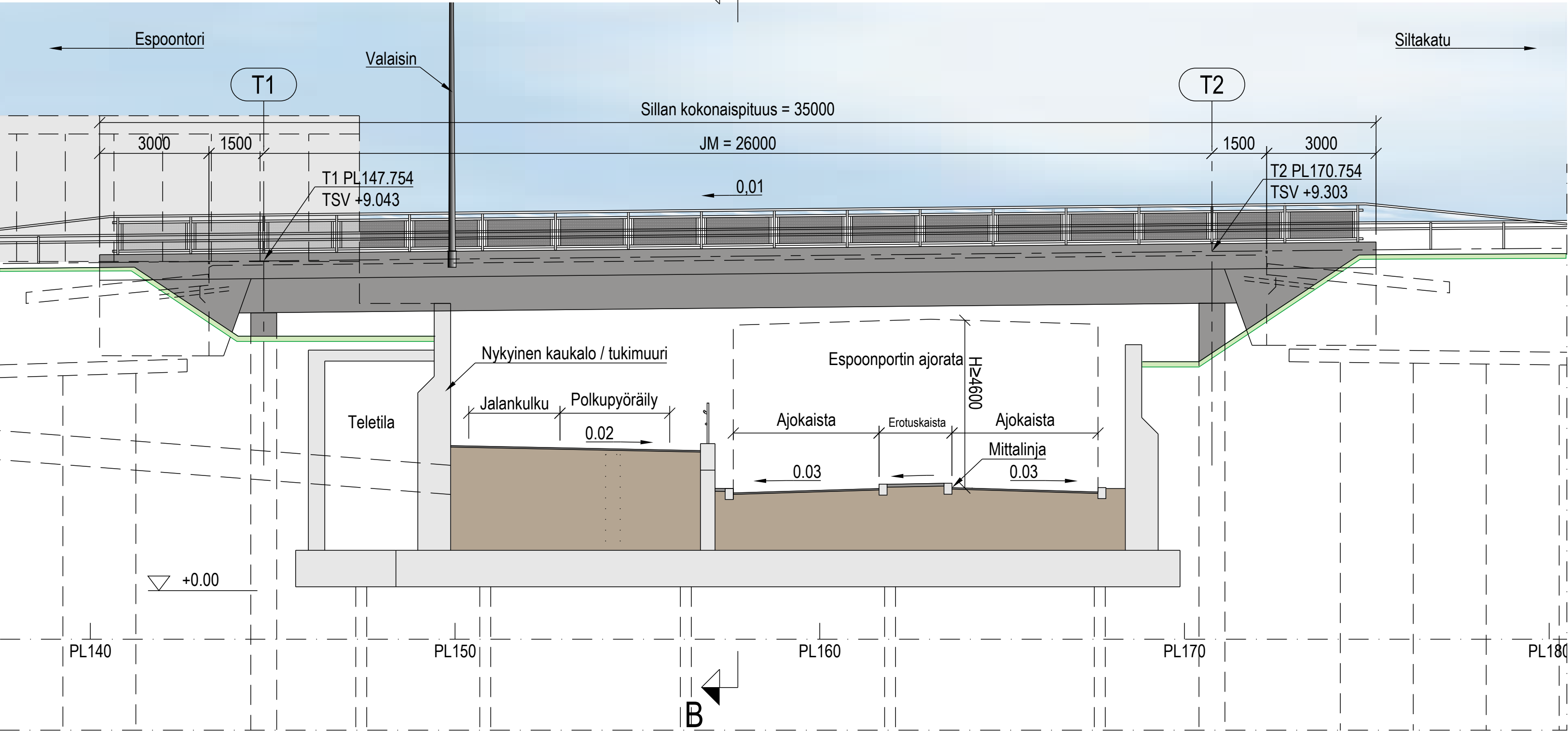
SIVUKUVA A - A 1:100
