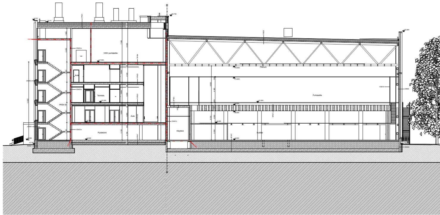
Leikkaus 340
