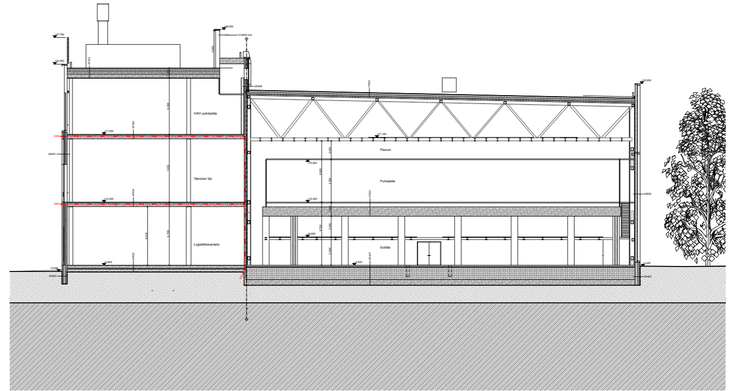
Leikkaus 380
