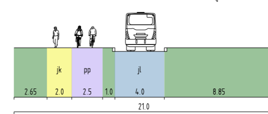
SALINPELLONTIE, LEIKKAUS C - C
