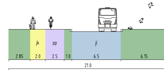
SALINPELLONTIE, LEIKKAUS B - B
