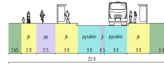
SALINPELLONTIE, LEIKKAUS D - D
