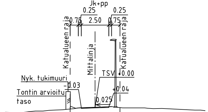
Kalevalantie TYYPPIPOIKKILEIKKAUS A-A 1:200
