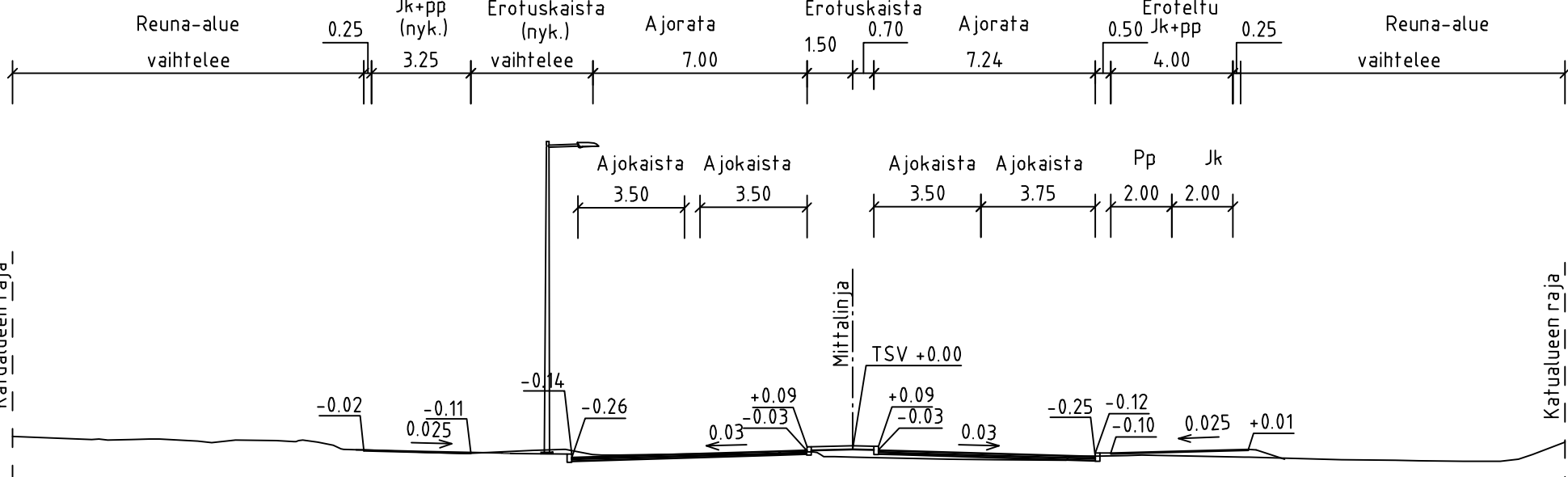
Kalevalantie TYYPPIPOIKKILEIKKAUS A-A 1:200
