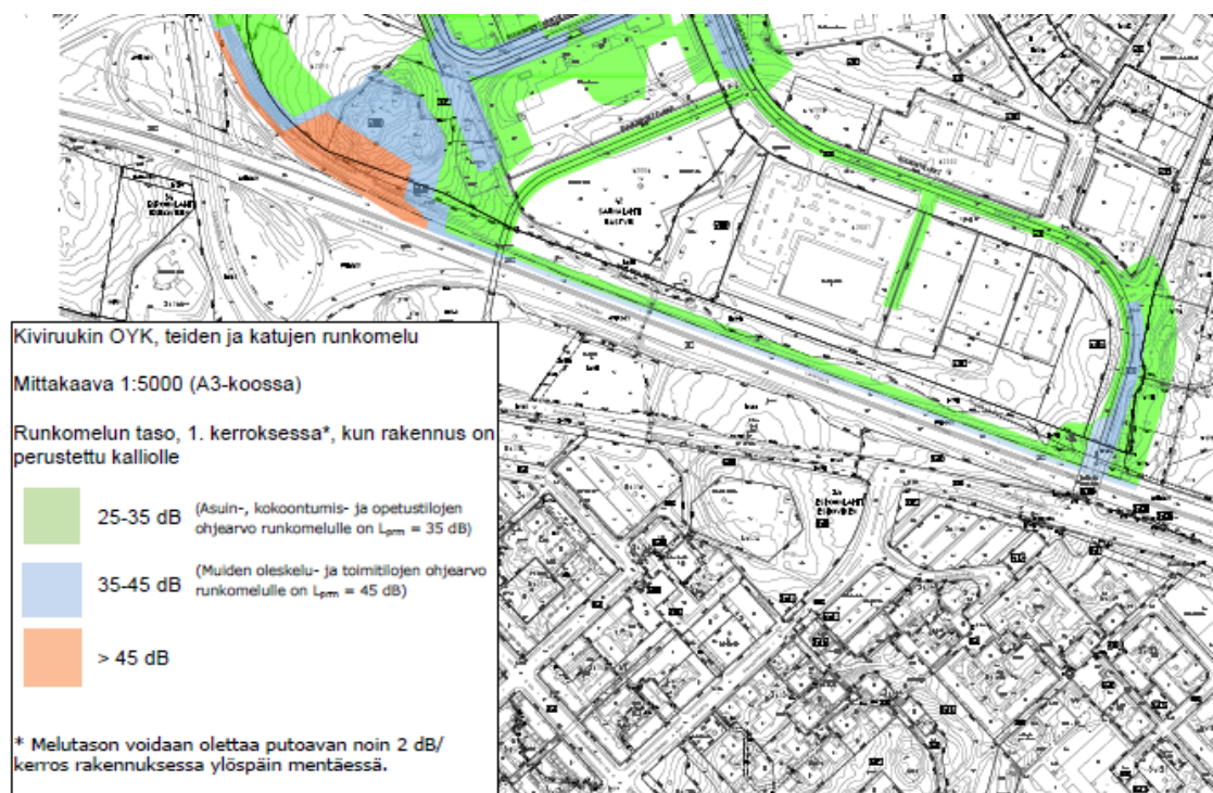
Kuva: Teiden ja katujen runkomelu (Kiviruukin OYK alue, Espoon kaupunki, Selvitys liikenteen aiheuttaman tärinän ja runkomelun vaikutuksista, Ramboll 2019).
