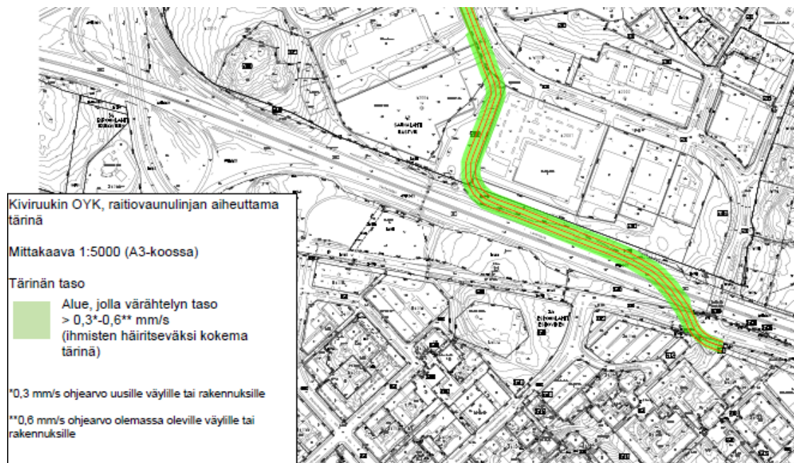
Kuva: Raitiovaunulinjan aiheuttama tärinä (Kiviruukin OYK alue, Espoon kaupunki, Selvitys liikenteen aiheuttaman tärinän ja runkomelun vaikutuksista, Ramboll 2019).
