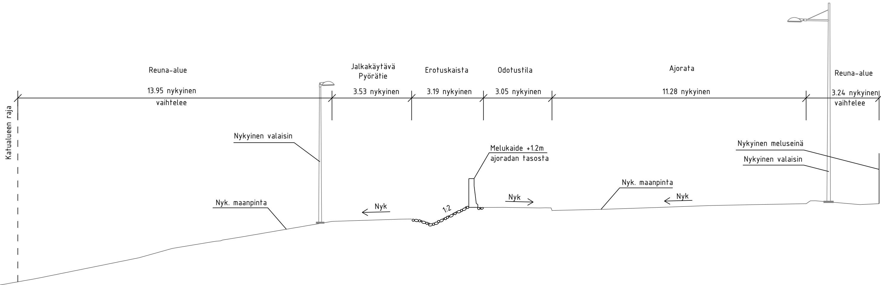
TYYPPIPOIKKILEIKKAUS A-A 1:100
