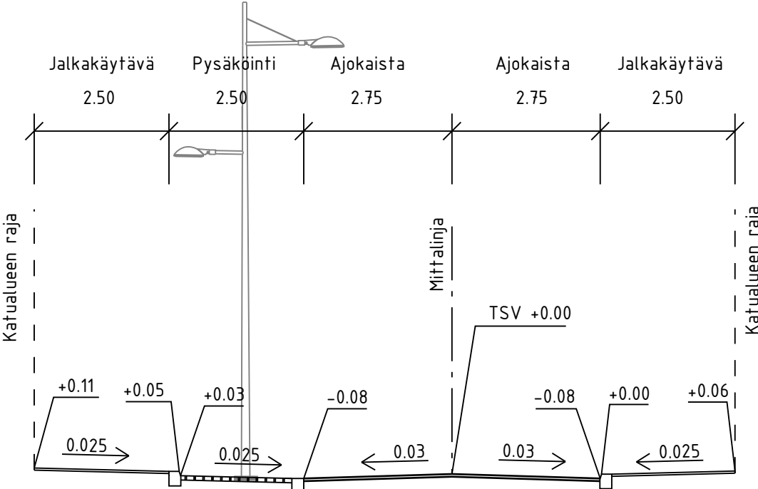
TYYPPIPOIKKILEIKKAUS A-A 1:100
