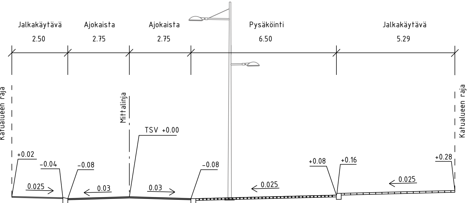
TYYPPIPOIKKILEIKKAUS B-B 1:100
