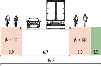
RUUTIKUJA, LEIKKAUS C - C
