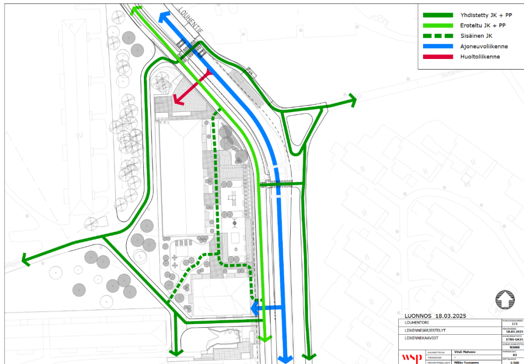
Korttelisuunnitelman liikennekaavio.
