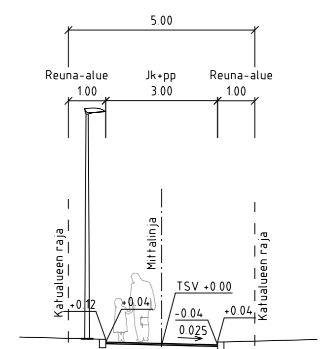
VÄLIKALLIONKUJA Jk+pp-tie TYYPPIPOIKKILEIKKAUS D-D 1:100
