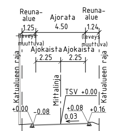
TYYPPIPOIKKILEIKKAUS B-B 1:200
