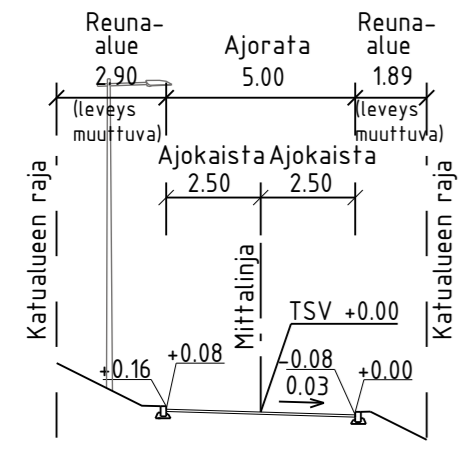
TYYPPIPOIKKILEIKKAUS A-A 1:200
