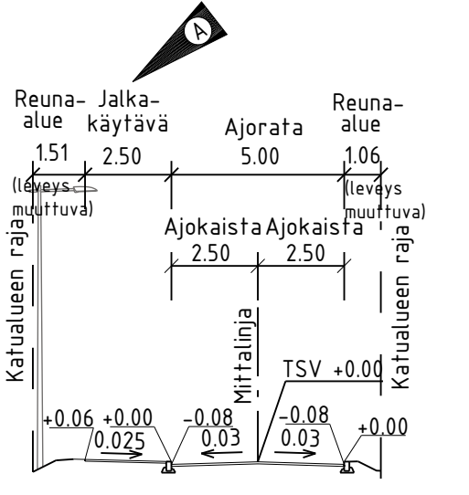
TYYPPIPOIKKILEIKKAUS A-A 1:200
