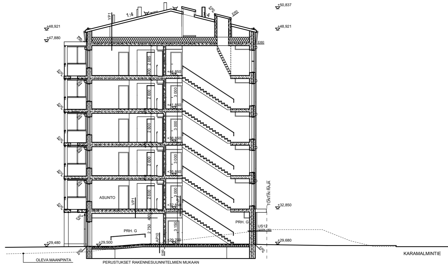
KIPSIMESTARI, LEIKKAUS G - G
