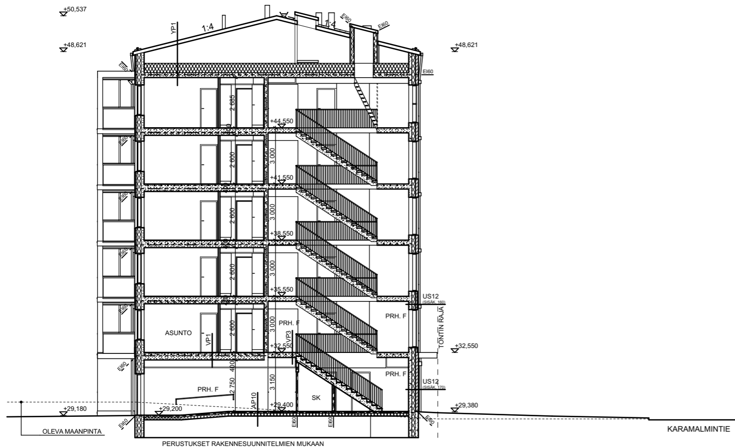
KIPSIMESTARI, LEIKKAUS F - F
