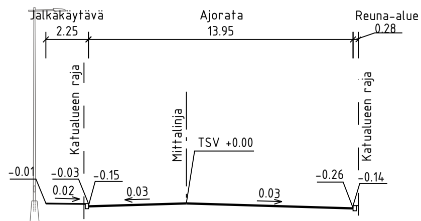
TYYPPIPOIKKILEIKKAUS A-A 1:200
