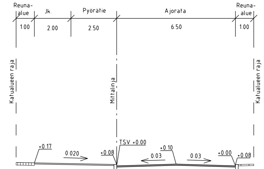
KOTKAPOLKU TYYPPIPOIKKILEIKKAUS A-A 1:100
