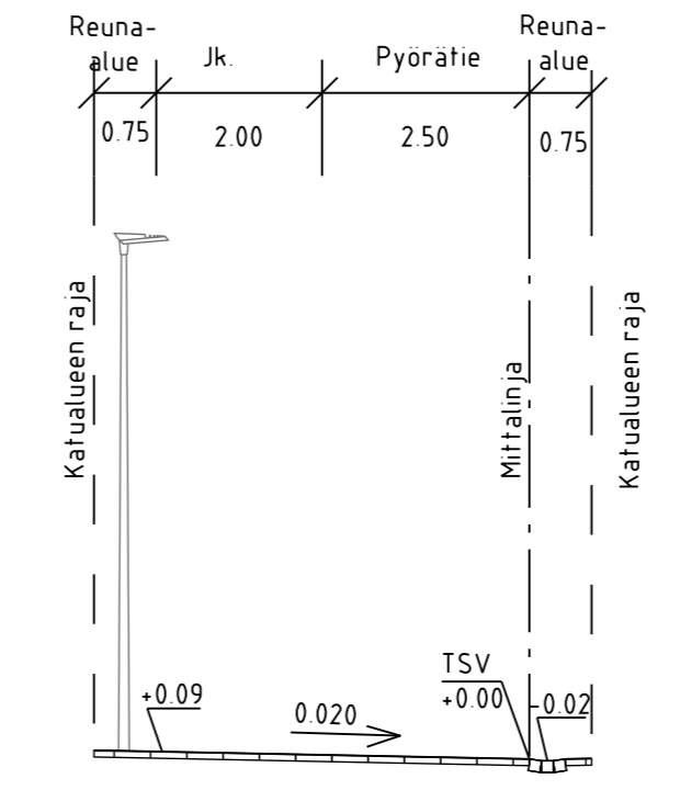
KOTKAPOLKU TYYPPIPOIKKILEIKKAUS B-B 1:100
