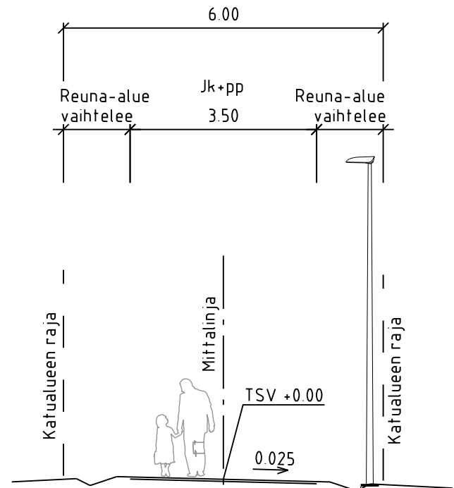
TYYPPIPOIKKILEIKKAUS A-A 1:100
