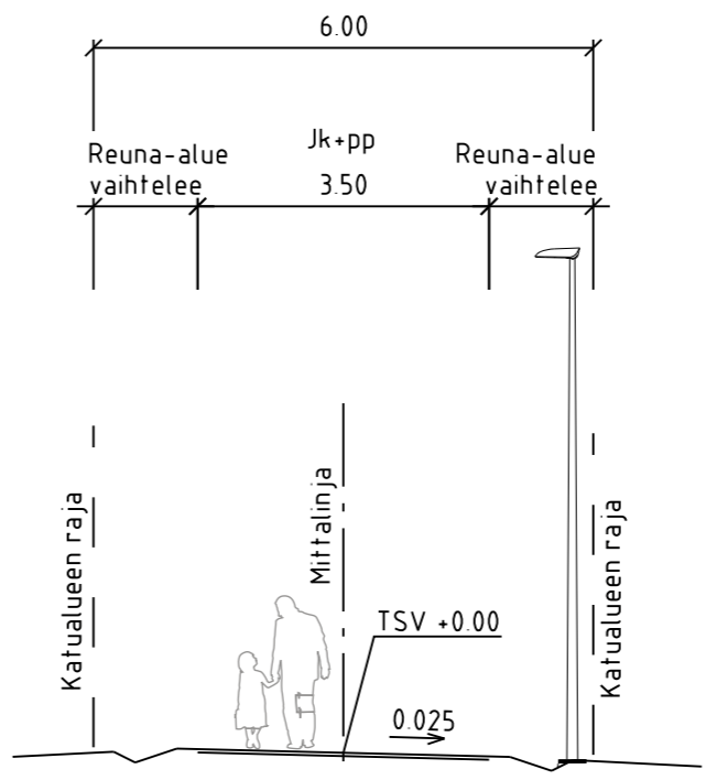
TYYPPIPOIKKILEIKKAUS A-A 1:100
