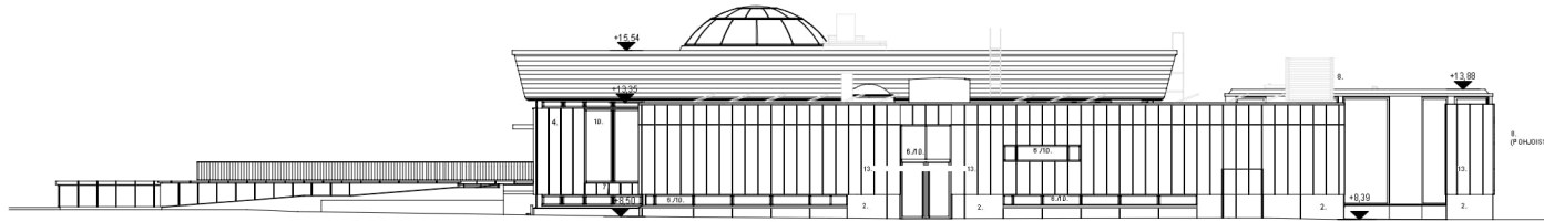
JULKISIVU ITÄÄN
