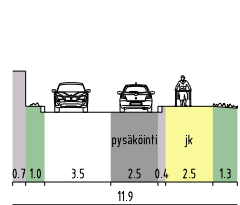
TAMARA BRUUNIN KATU, LEIKKAUS P - P
