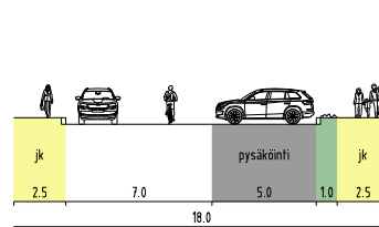
ALOITTAJANKATU, LEIKKAUS H - H
