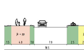
TAMARA BRUUNIN KATU, LEIKKAUS P - P
