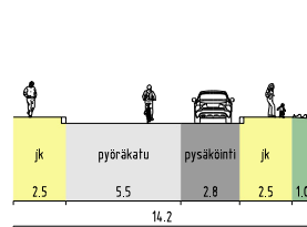
LILLBASSINKATU, LEIKKAUS F - F
