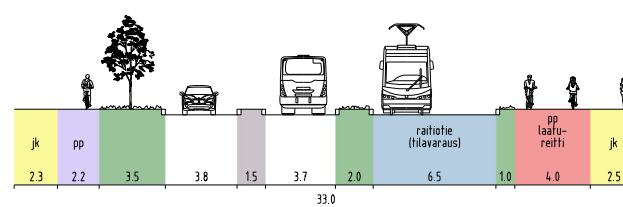
VANTINMÄENTIE, LEIKKAUS I - I
