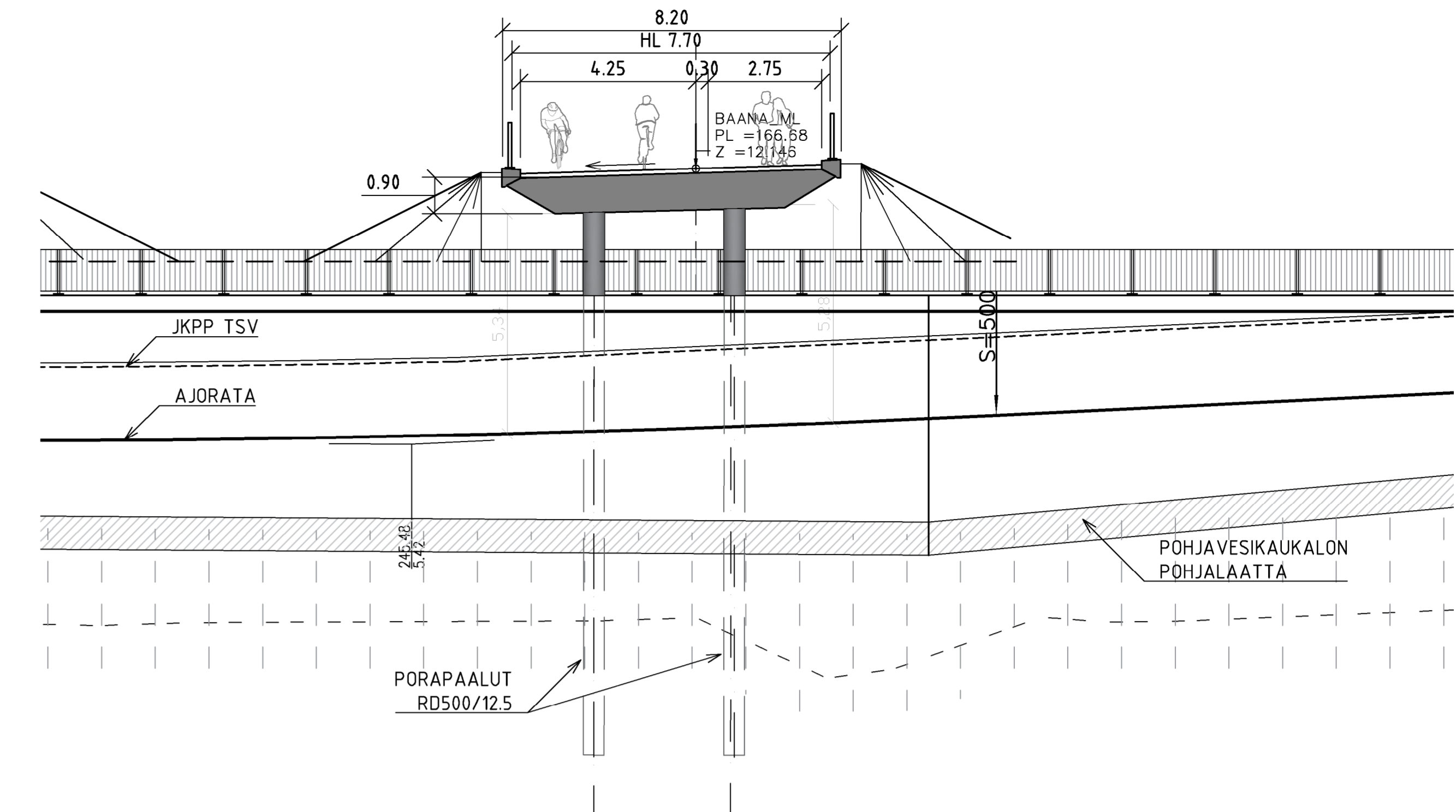
POIKKILEIKKAUS A-A 1:100
