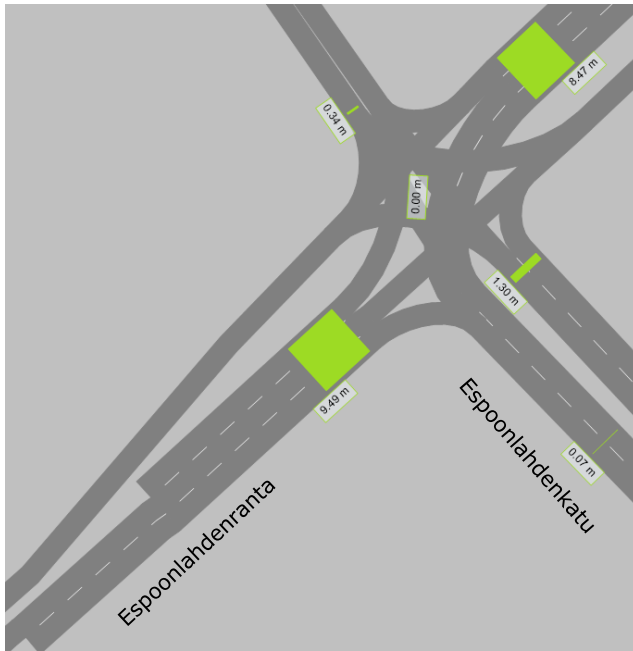
Kuva 27. Espoonlahdenrannan keskimääräinen jononpituus (vasen) ja hetkittäinen maksimijononpituus (oikea). Nykyinen oikealle kääntymiskaista, AHT.
