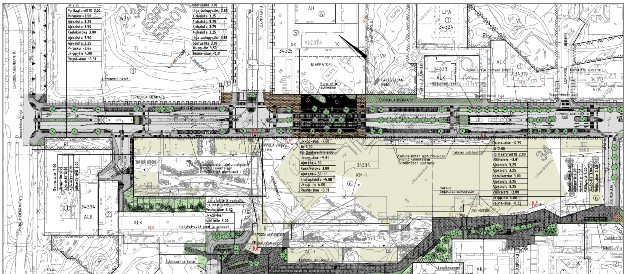
Kuva 5. Espoonlahden keskuksen katusuunnitelman kostepiirustus (Ramboll 8.7.2016).
