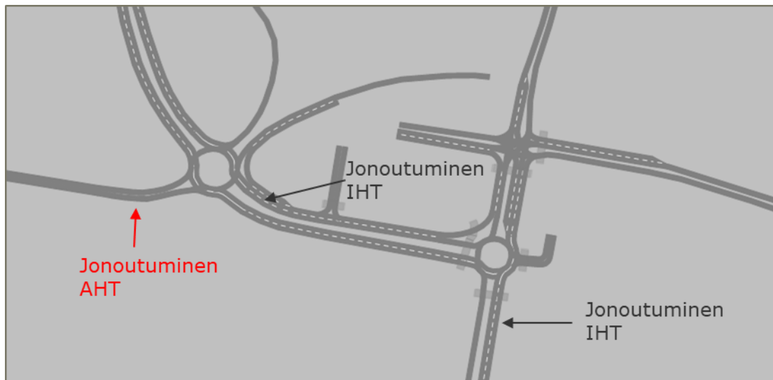
Kuva 37. Kivenlahden jonoutuneet suunnat oletusverkolla.
