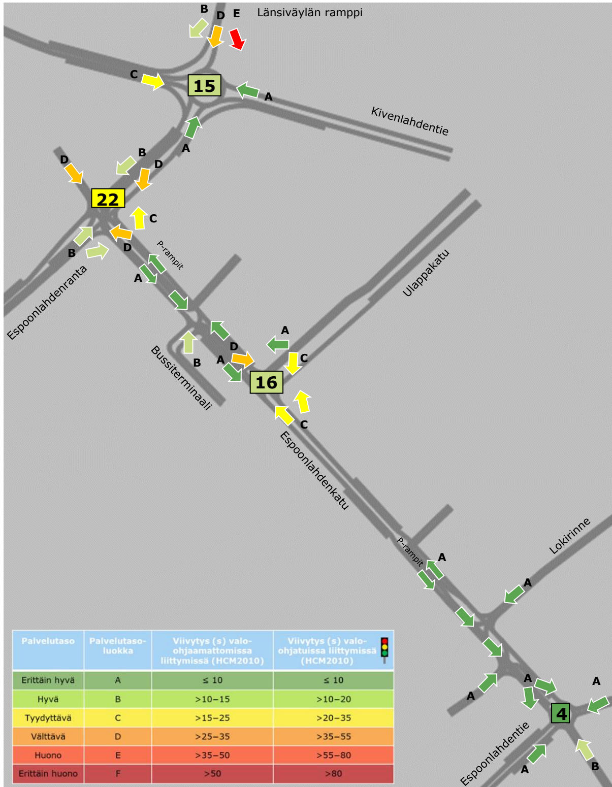
Kuva 24. Espoonlahden keskuksen liittymien keskimääräiset viivytykset sekunteina sekä suuntaakohtaiset palvelutasot, kiertoliittymävaihtoehdon IHT.
