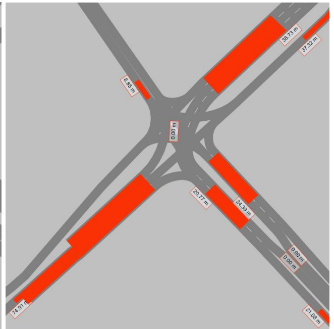
Kuva 27. Espoonlahdenrannan keskimääräinen jononpituus (vasen) ja hetkittäinen maksimijononpituus (oikea). Nykyinen oikealle kääntymiskaista, AHT.
