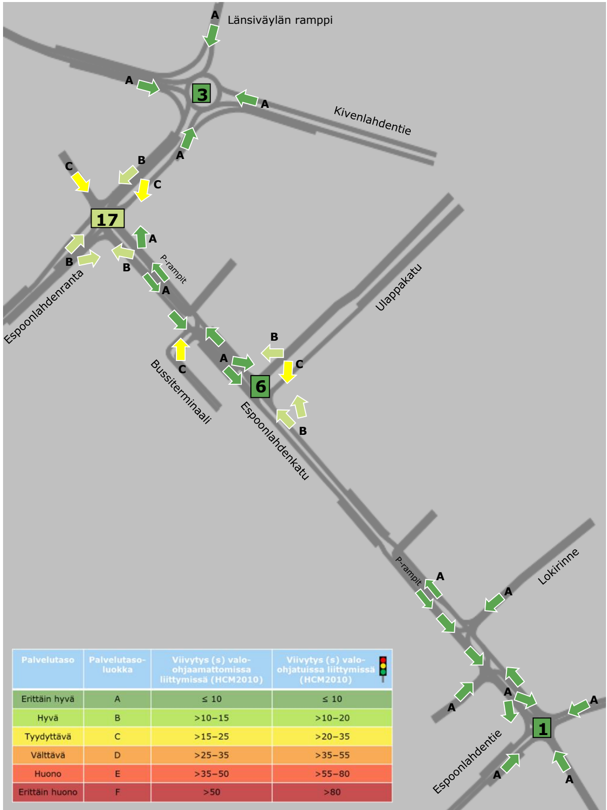
Kuva 18. Espoonlahden keskuksen liittymien keskimääräiset viivytykset sekunteina sekä suuntakohtaiset palvelutasot, nelihaaravaihtoehdon AHT.
