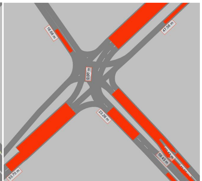
Kuva 28. Espoonlahdenrannan keskimääräinen jononpituus (vasen) ja hetkittäinen maksimijononpituus (oikea). Nykyinen oikealle kääntymiskaista, IHT.
